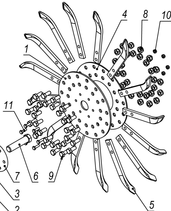
РБА-6Н_02.04.000-01 Секция зубьев
