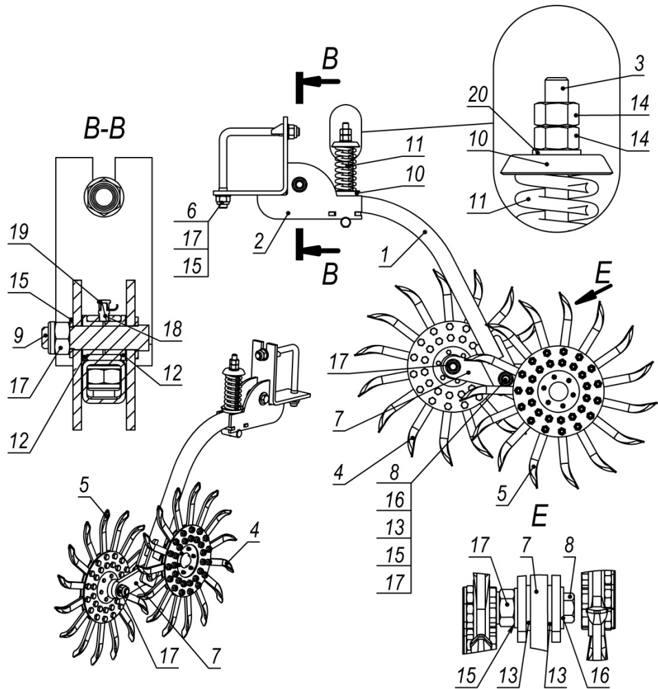
6. Секція робоча РБА-6Н_02.00.000 (мал.4).
