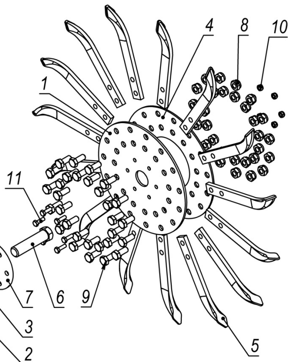
РБА-6Н_02.04.000-01 Секция зубьев
