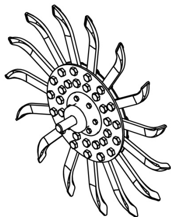
РБА-6Н_02.04.000-01 Секция зубьев
