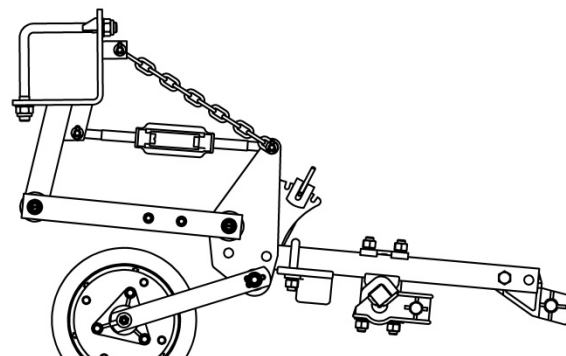
КРНА-5.6Н_02.00.000-02 Секция рабочая
