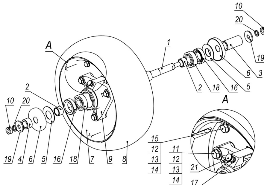
КРНА-5.6Н_02.04.000-01 Колесо
