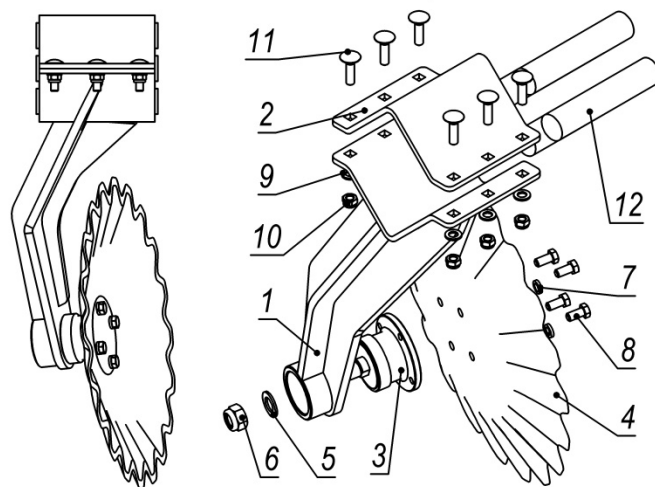
БДАД-6ПГ_07.00.000 Стойка задняя (Остальное БДАД-6ПГ_06.00.000)
