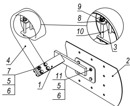
БДА-4ПЦ_08.00.000-01 Щиток
