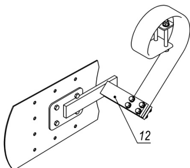
БДА-4ПЦ_08.00.000-01 Щиток
