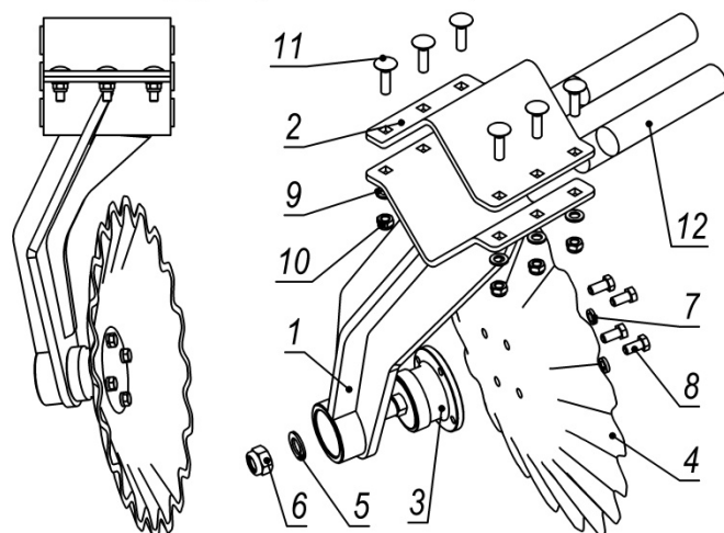
БДАД-6ПГ_07.00.000 Стойка задняя (Остальное БДАД-6ПГ_06.00.000)
