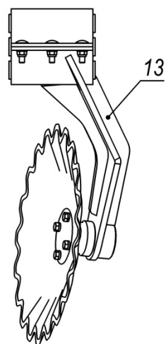
БДАД-6ПГ_07.00.000 Стойка задняя (Остальное БДАД-6ПГ_06.00.000)
