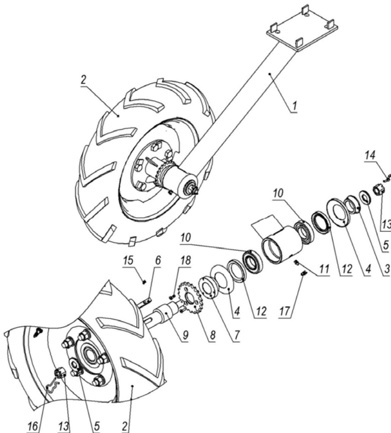
Малюнок 5 – Колесо опорно-привідне.
