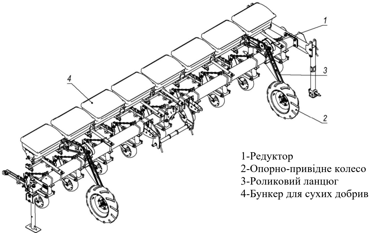
Малюнок 3.2 – Культиватор із системою внесення рідких
