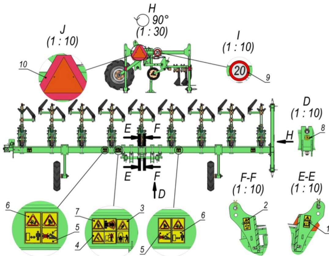
Малюнок 1 – Розташування попереджувальних знаків КРНА-5,6-01Н
