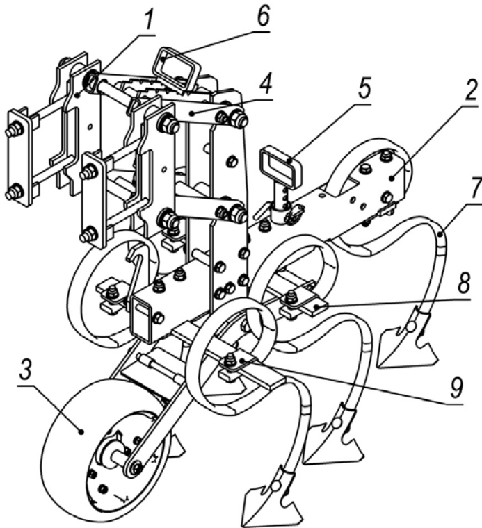
Малюнок 4 – Робоча секція навісного культиватора.
