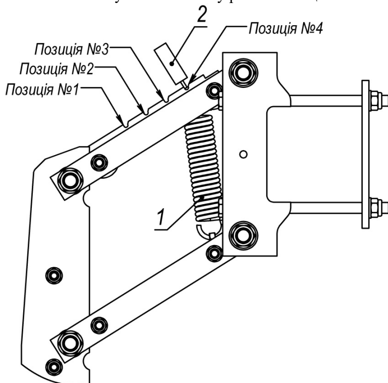
Малюнок 8 – Регулювання тиску робочої секції.
