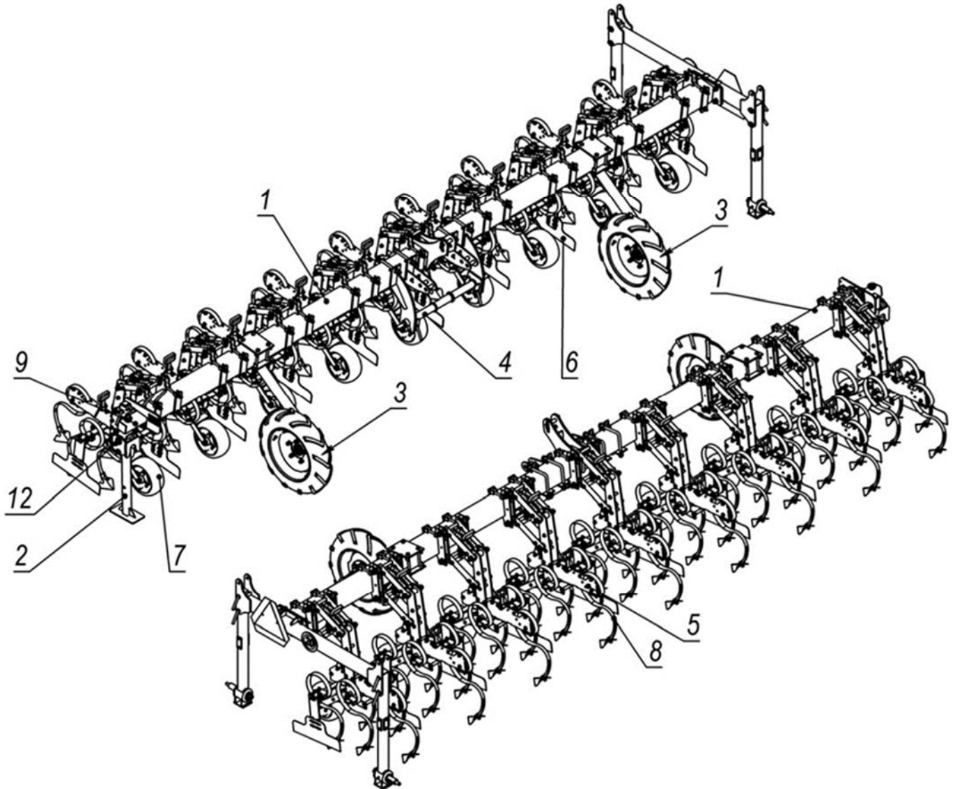
Малюнок 3 – Міжрядковий культиватор КРНА-5,6-01Н .
