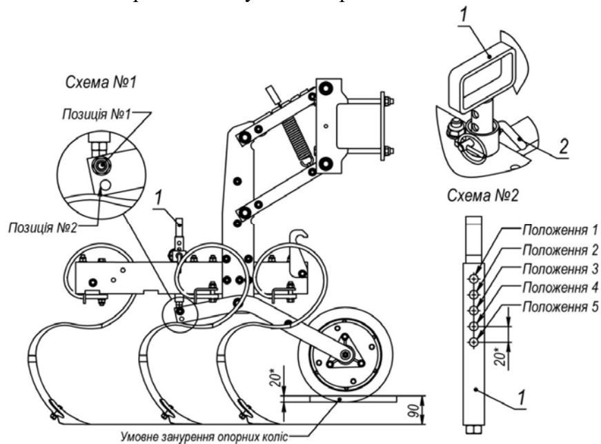
Малюнок 7 – Робоча секція міжрядкового культиватора.
